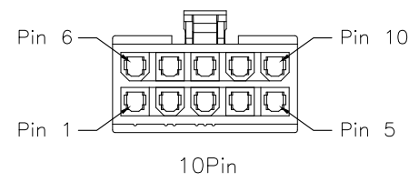
2~24Pin 防呆示意图(Ref.)
