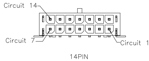
14PIN
