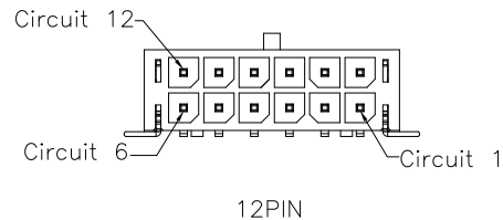
12PIN
