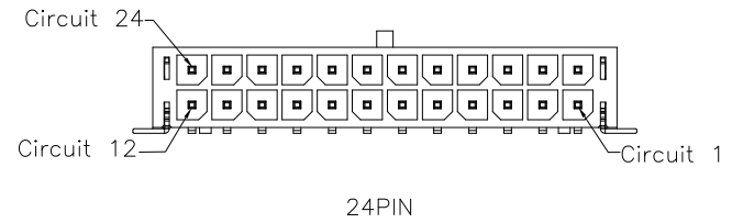
24PIN
