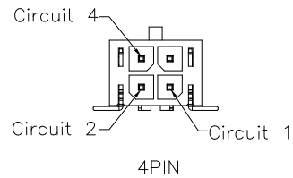
4PIN
