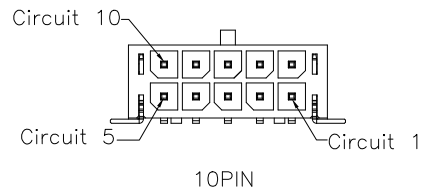
10PIN
