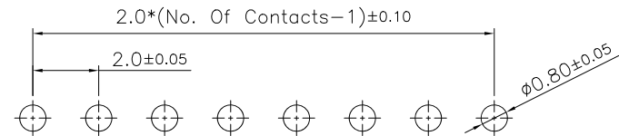
P.C.B Layout
