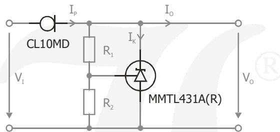
Fig. 3 Spannungsversorgung mit geringem Bauteilbedarf für µController und andere Schaltungen mit niedrigem Eingangstrom
