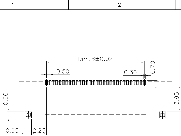
P.C.B LAYOUT
